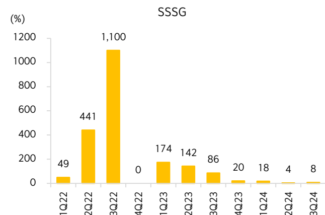
Fig. 4: SSSG
